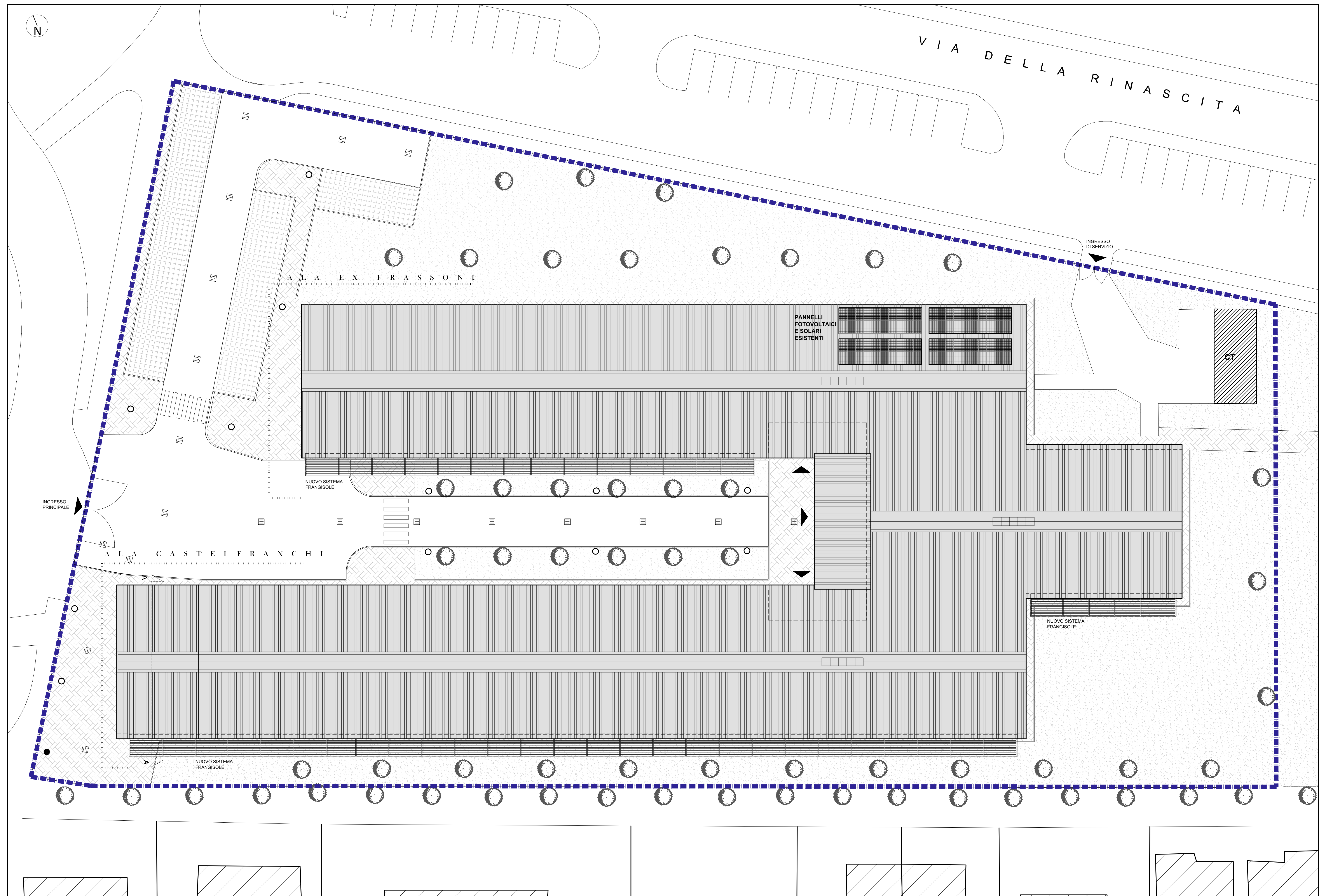
PLANIMETRIA GENERALE - PIANTA COPERTURA
